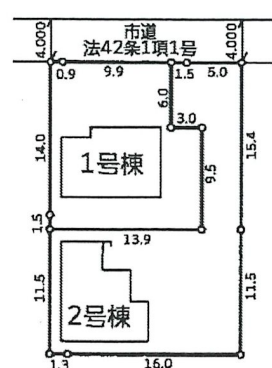
【図面配置】
